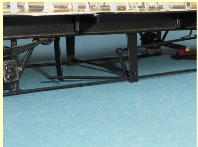
Détail Frein 2
